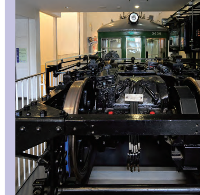
デハ3450形車両の実車を分解展示。構造や操作が分かる。
